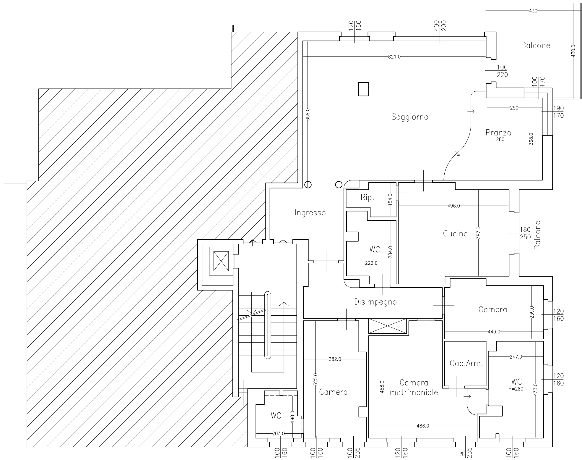
PIANTA PIANO PRIMO - H=290 stato di fatto
